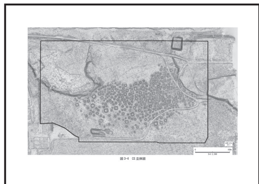
(3) レーザー計測による地形図
